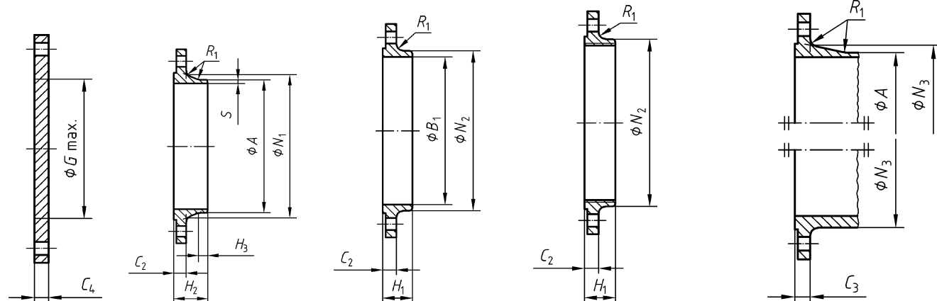
h) Type 05 i) Type 11 j) Type 12 k) Type 13 l) Type 21
